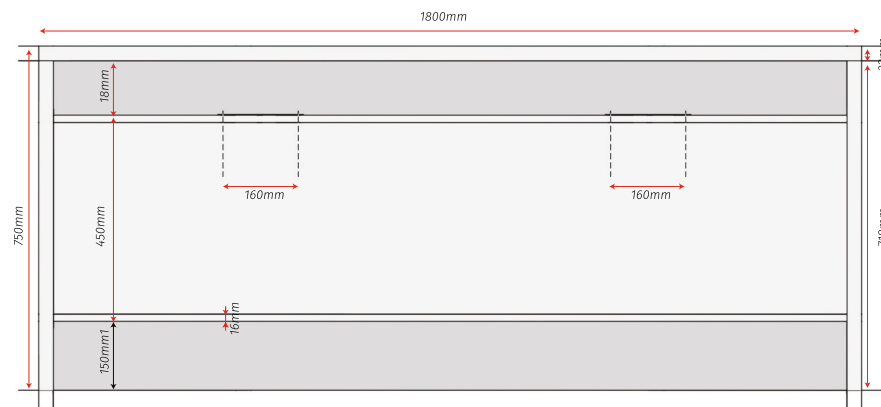
Вид спереди
