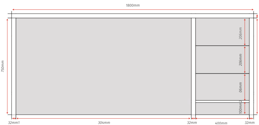
Вид сзади
